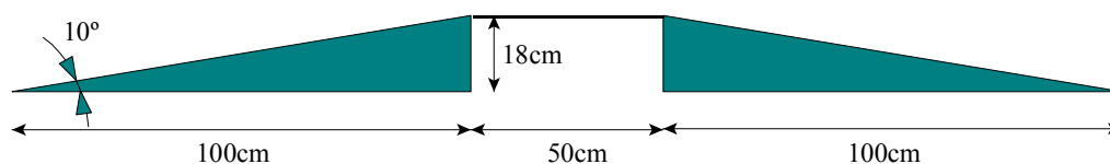
Figura 2. Vista lateral del puente (dimensiones aproximadas).
